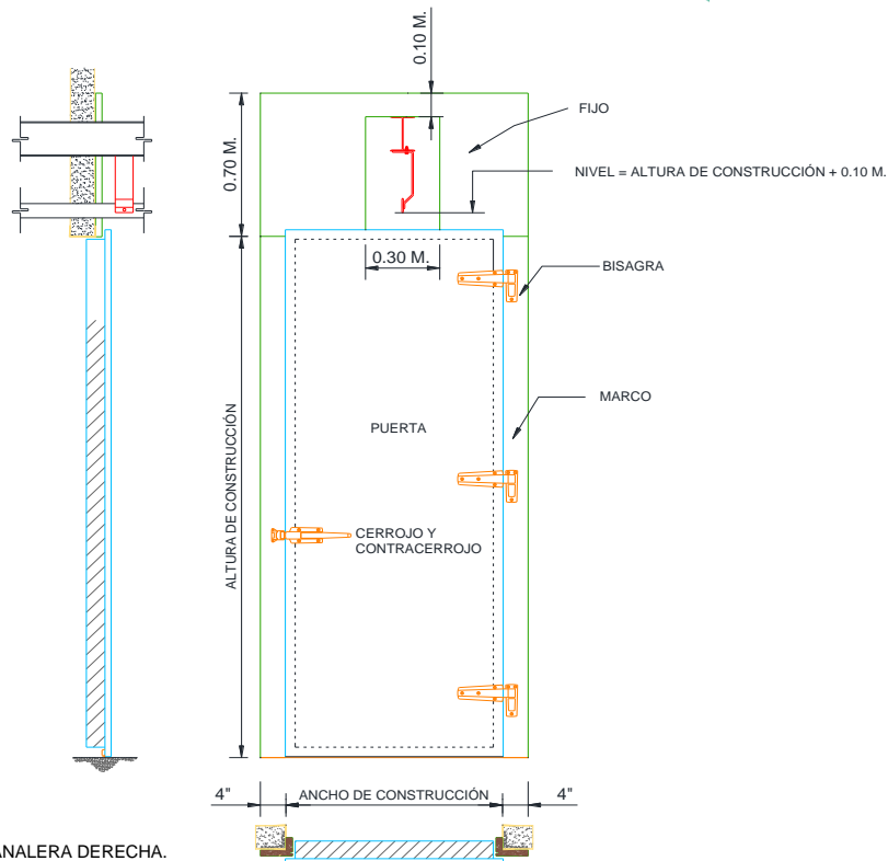
JUN-2020. IMAGEN: PUERTA ABATIBLE CANALERA DERECHA.
