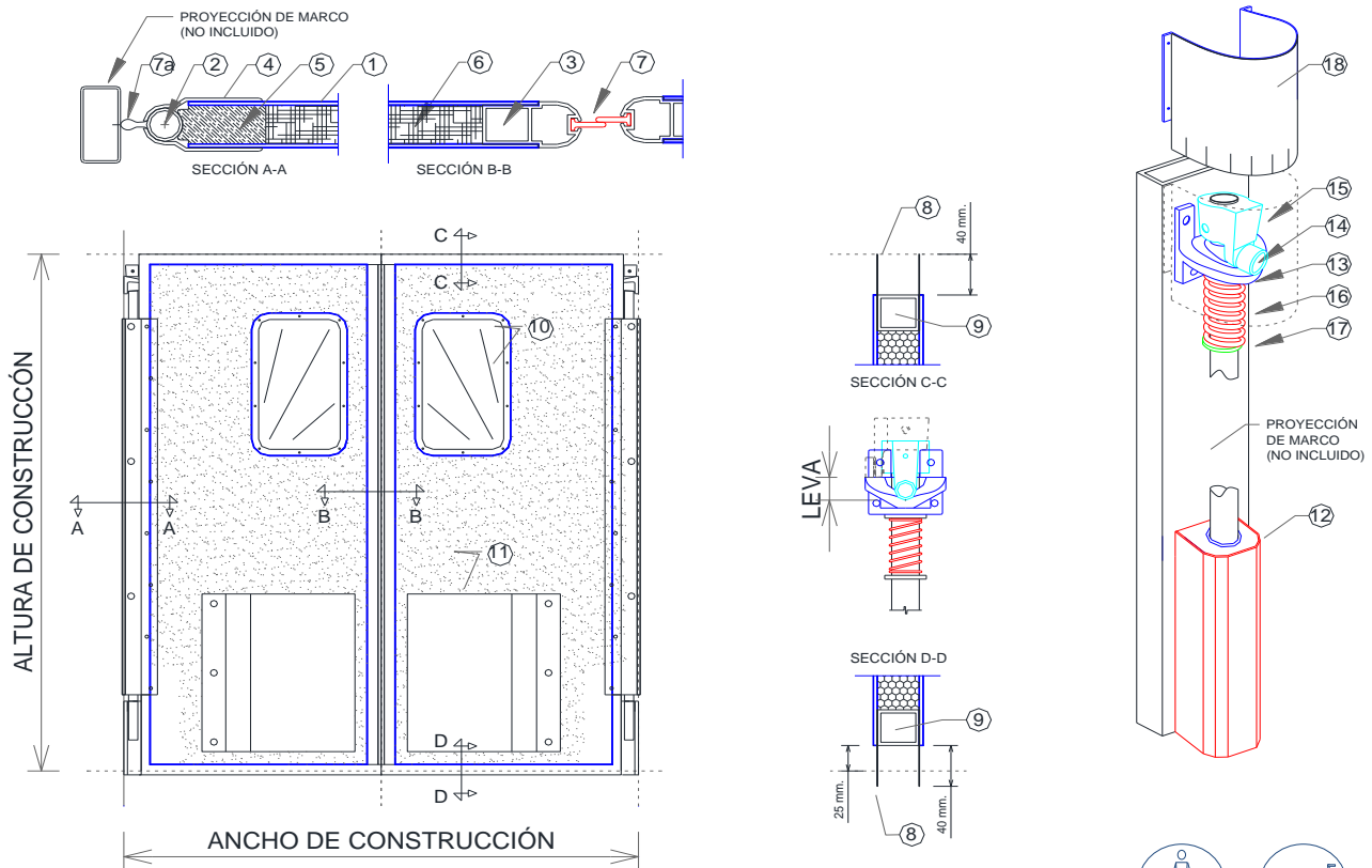
JUN-2020 VISTA PUERTA UNI-SWING DOBLE
