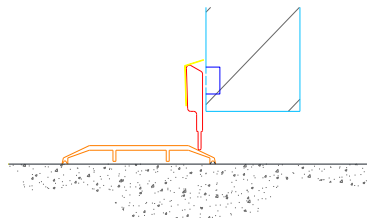
Detalle Arrastre
